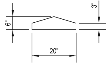
COLUMN CAP
